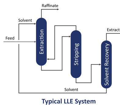
Typical LLE System
